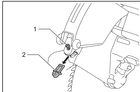
► 1. Screw 2. Lens
