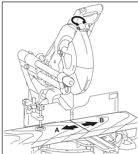
► 1. Clé hexagonale
